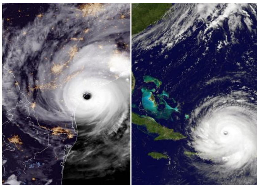
ハーヴィ (左) とアーマの衛星写真
